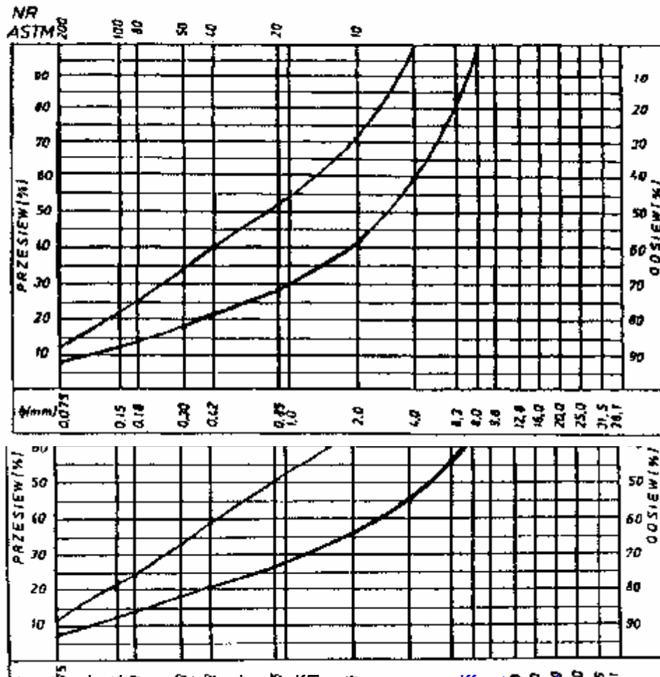
Rys. 2. Krzywe graniczne uziarnienia mieszanki mineralnej 0,16, 0,12,8 mm do warstwy ścieralnej z betonu asfaltowego dla KR 1-2
