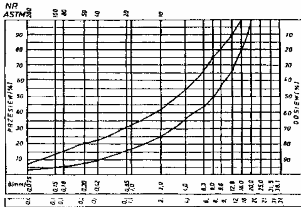
Rys. 11. Krzywe graniczne uziarnienia mieszanki mineralnej 0, 25 mm do warstwy , wyrównawczej i z betonu asfaltowego dla KR 3-6
