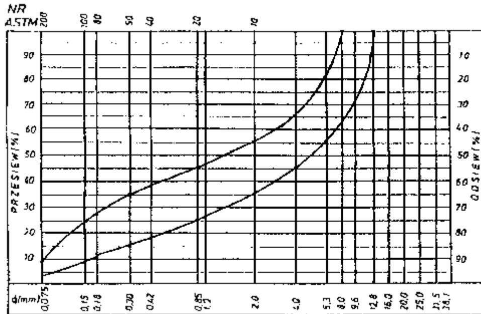
Rys. 10. Krzywe graniczne uziarnienia mieszanki mineralnej 0, 12,8 mm do warstwy , wyrównawczej z betonu asfaltowego dla KR 1-2
