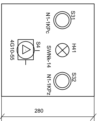
Pokrywa skrzynek typu Z2 Elewacja
