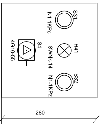
Pokrywa skrzynek typu ZZ Elewacja
