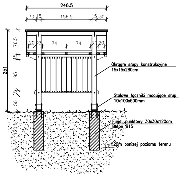
PRZEKRÓJ PODŁUŻNY
