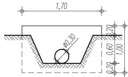
ŚCIANKI CZOŁOWE PRZEPUSTU
