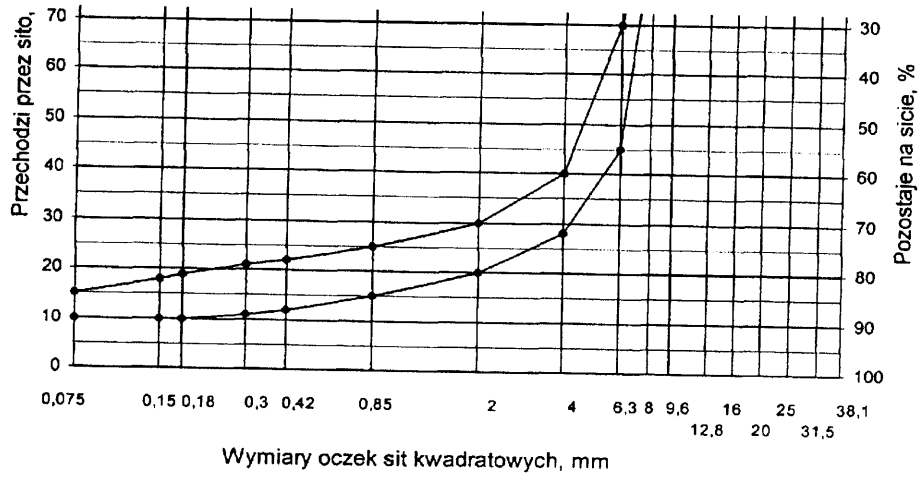
Rys. 2. Krzywe graniczne uziarnienia mieszanki mineralnej SMA od 0 do 8 mm do warstwy ścieralnej nawierzchni drogi o obciążeniu ruchem KR1 lub KR2
