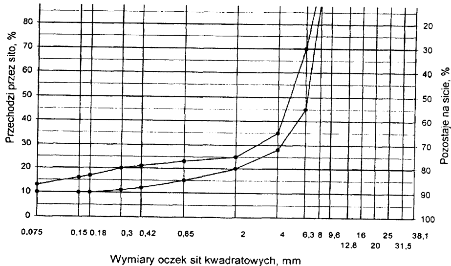
Rys. 7. Krzywe graniczne uziarnienia mieszanki mineralnej SMA od 0 do 8 mm do warstwy ścieralnej nawierzchni drogi o obciążeniu ruchem od KR3 do KR6
