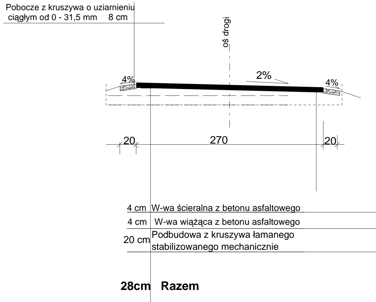
PRZEKRÓJ POPRZECZNY DROGOWY Rys. nr 1 odcinek w km 0+000 - 0+507
