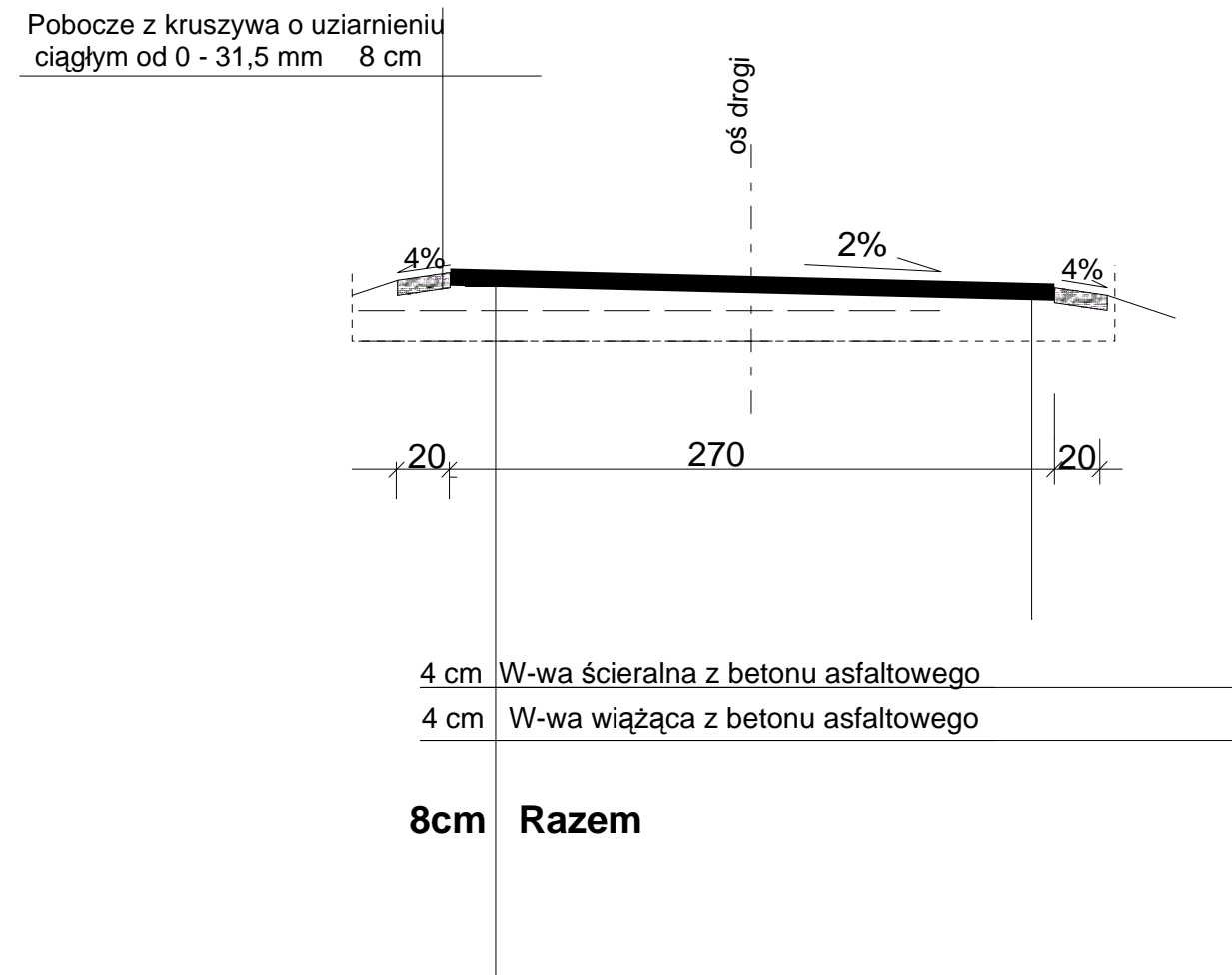
PRZEKRÓJ POPRZECZNY DROGOWY Rys. nr 2 odcinek w km 0+507 - 0+816
