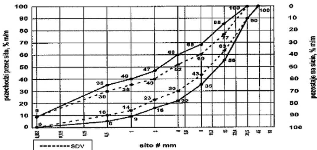
Krzywe graniczne uziarnienia mieszanki kruszywa niezwiązanego 0/31,5 mm do warstw podbudowy zasadniczej.
